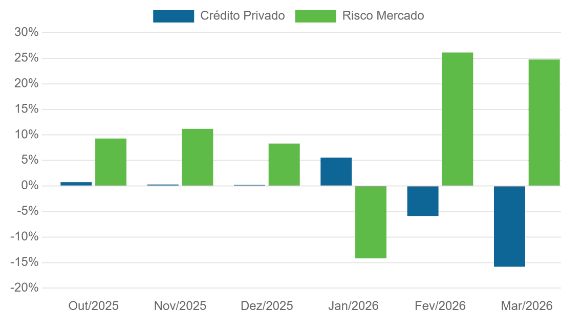
PnL Mensal (Alfa %CDI)
